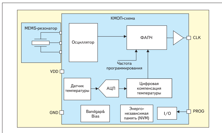
Рис. 1. Структурная схема программируемого МЭМС-генератора
