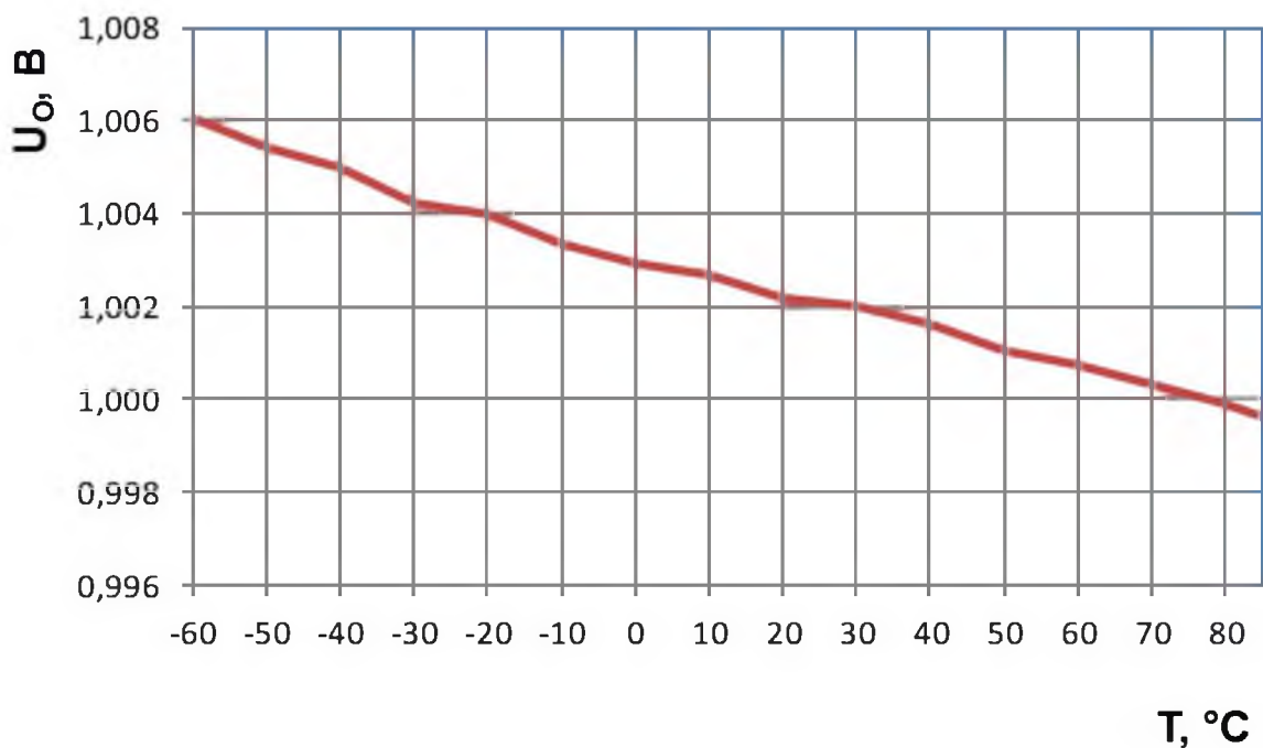
Рисунок 6 – Зависимость минимального выходного напряжения U_o микросхемы 1309ЕР1Т от температуры корпуса при U_i = 2 В, I_o = 10 мА
