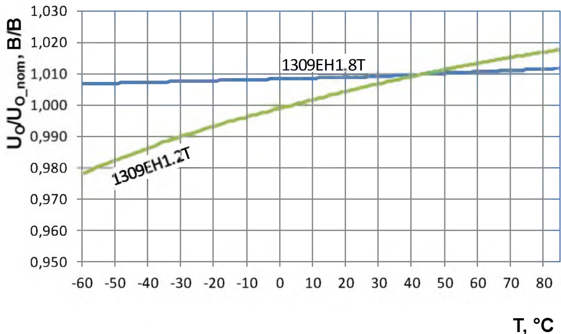
Рисунок 5 – Зависимость выходного напряжения U_o (приведенного к выходному напряжению номинальному U_{o\_ном} ) от температуры корпуса при U_i = U_{i\ min} В, I_o = 10 мА
