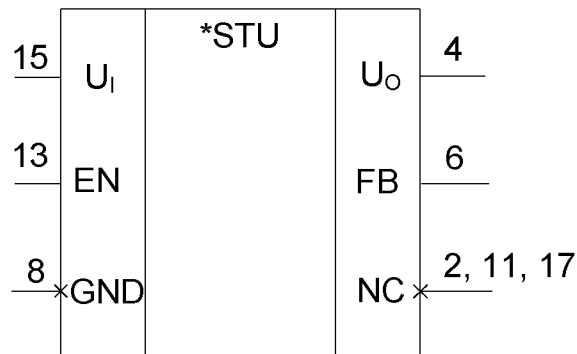
Рисунок 1 – Условное графическое обозначение
