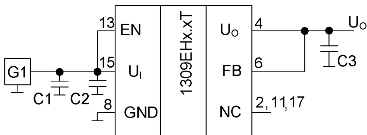
Рисунок 3 – Типовая схема включения микросхемы 1309EP1Т с внешним делителем
