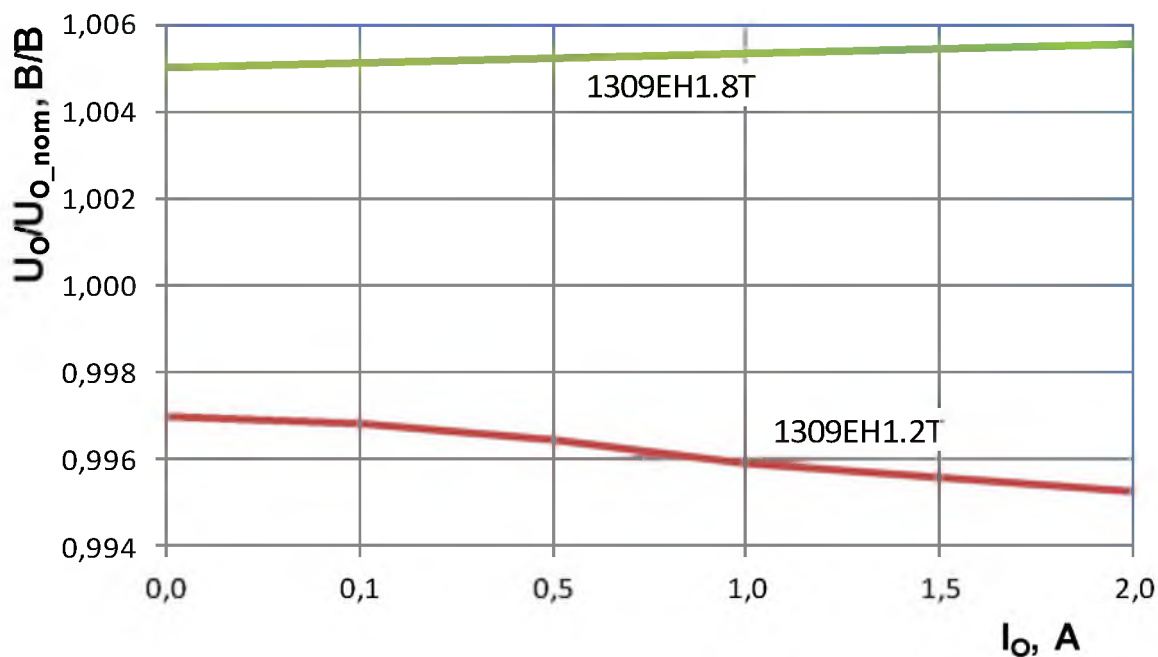
Рисунок 9 – Зависимость выходного напряжения U_o (приведенного к выходному напряжению номинальному U_{o\_nom} ) от тока нагрузки при U_i = 2,8 В для 1309ЕН1.2Т и U_i = 2,6 В для 1309ЕН1.8Т, T = 25 °С
