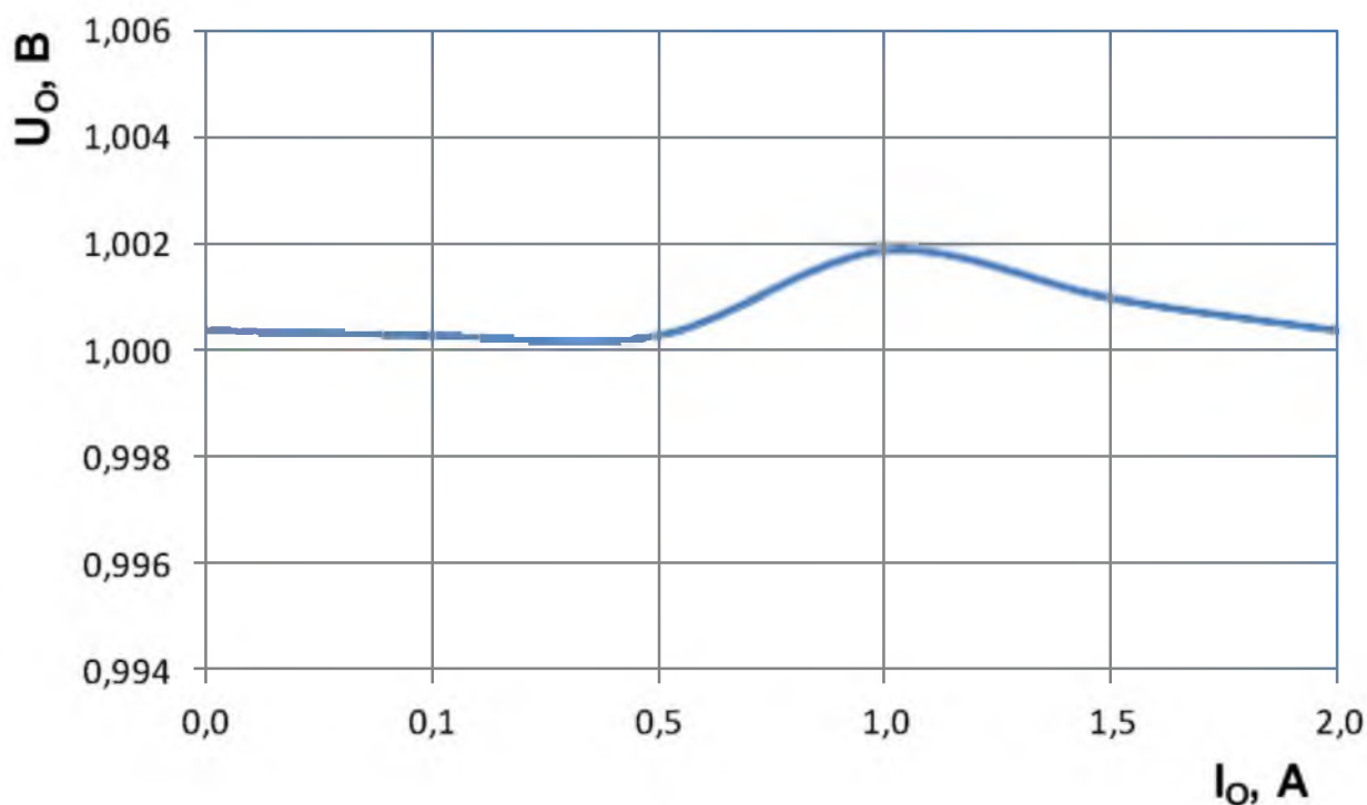
Рисунок 10 – Зависимость минимального выходного напряжения U_o микросхемы 1309ЕР1Т от тока нагрузки при U_i = 2,5 В, T = 25 °С
