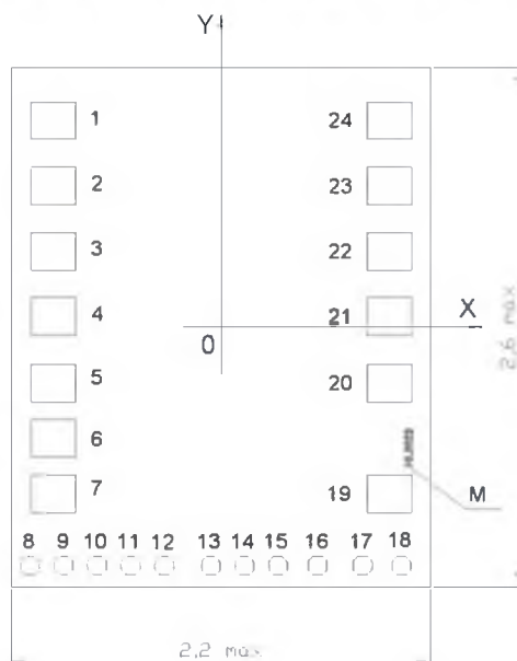
Рисунок 20 – Корпус 4116.8-3
