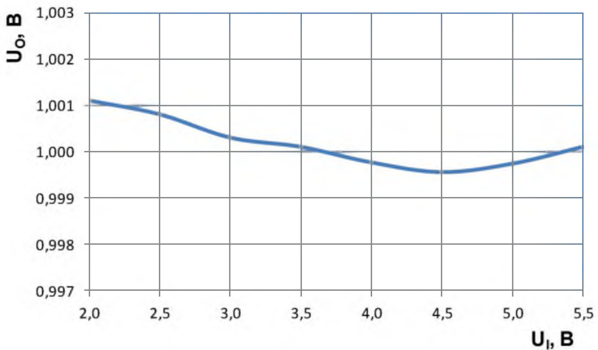
Рисунок 8 – Зависимость минимального выходного напряжения U_o микросхемы 1309EP1T от входного напряжения при I_o = 100 мА, T = 25 °С
