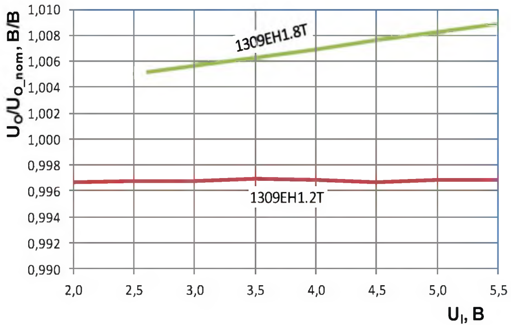
Рисунок 7 – Зависимость выходного напряжения U_o (приведенного к выходному напряжению номинальному U_{o\_ном} ) от входного напряжения при I_o = 100 мА, T = 25 °С
