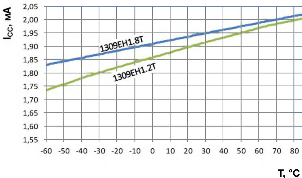
Рисунок 19 – Зависимость тока потребления I_{CC} от температуры при U_I = 5,5 В, I_O = 10 мА
