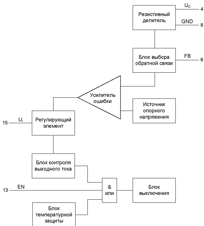
Рисунок 2 – Структурная блок-схема микросхемы
