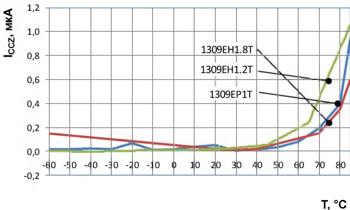
Рисунок 20 – Зависимость тока потребления в состоянии выключено I_{CCZ} от температуры корпуса
